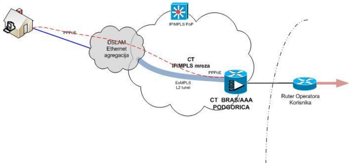
Slika 1. Način realizacije usluge veleprodajnog širokopojsnog pristupa za Internet uslugu na IP nivou korišćenjem ADSL tehnologije
