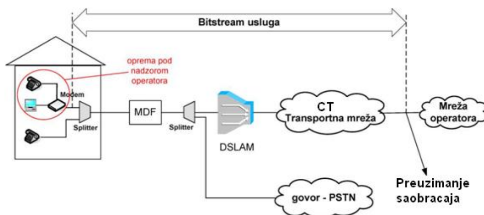
Slika 3. Koncept posebnog virtuelnog kanala za VoIP uslugu
