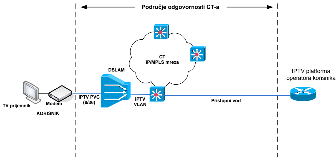
Slika 6. Realizacija posebnog virtualnog kanala za IPTV uslugu preko ADSL pristupa
